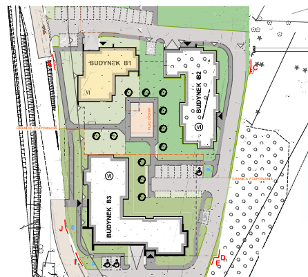
PLAN ZAGOSPODAROWANIA TERENU
